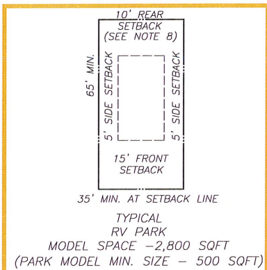
TYPICAL RV SPACES N.T.S.
