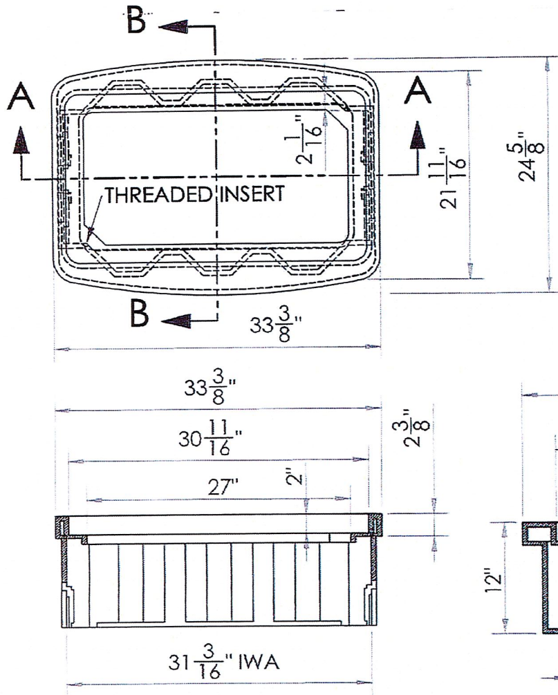
SECTION A-A SCALE 1 : 12
