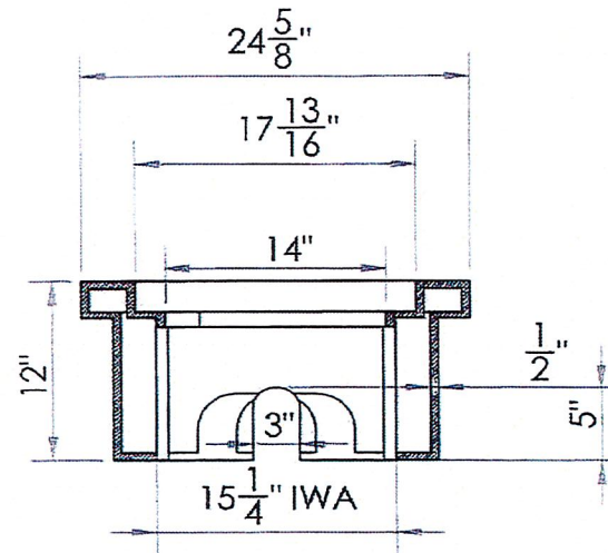
SECTION B-B SCALE 1 : 12
