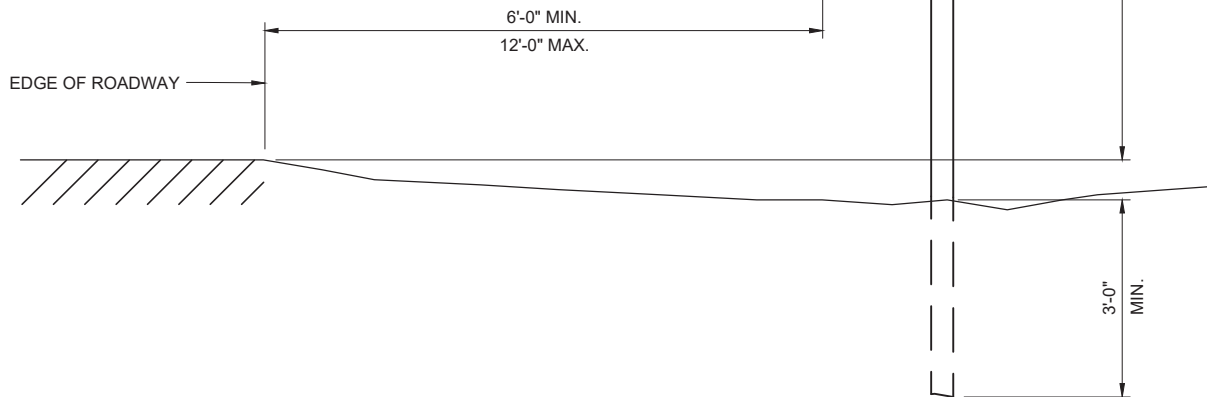
ELEVATION
